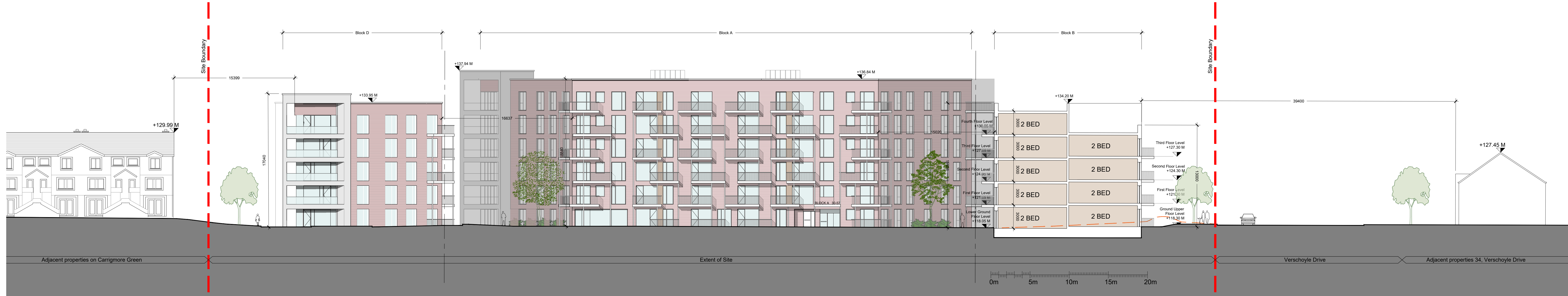
Section AA Scale: 1:200 @ A0
