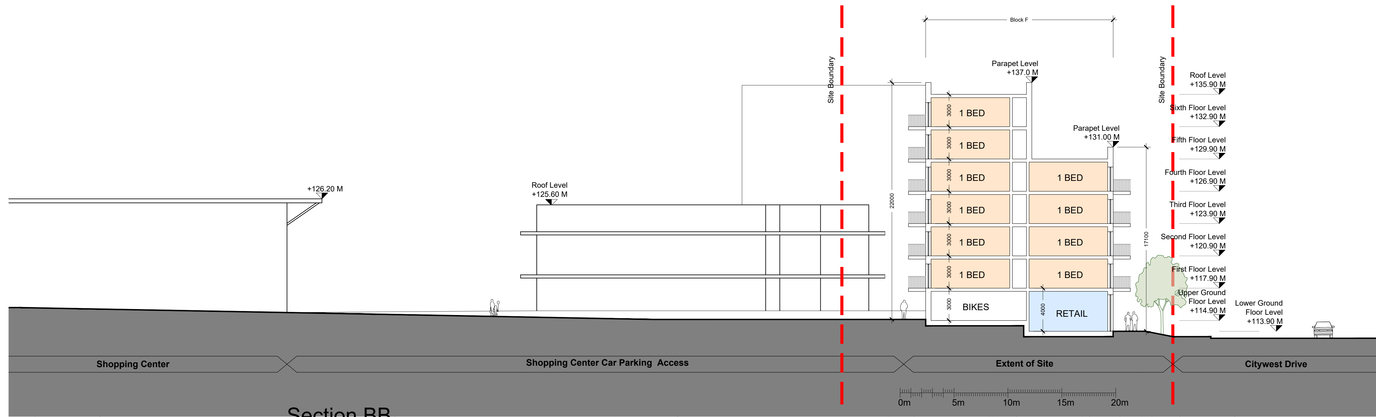
Section BB Scale: 1:200 @ A0
